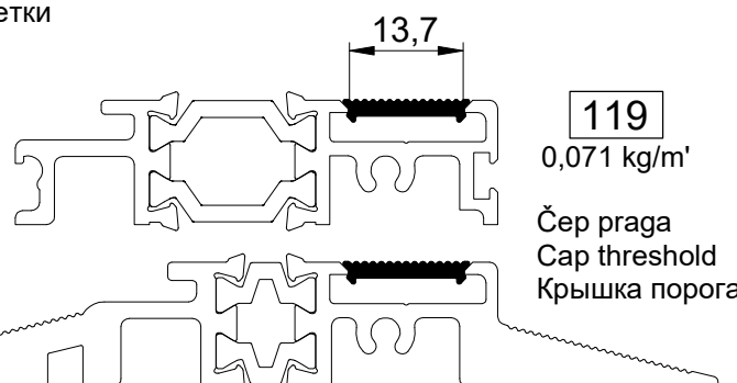
TM33 0,152 kg/m' Pogonska letva Mechanism rod Шток механизма
