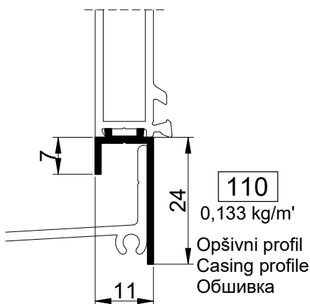
Profil za prihvatanje obloge Cladding mounting profile Профиль для приема облицовки
