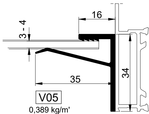
Profil za prihvatanje obloge Cladding mounting profile Профиль для приема облицовки
