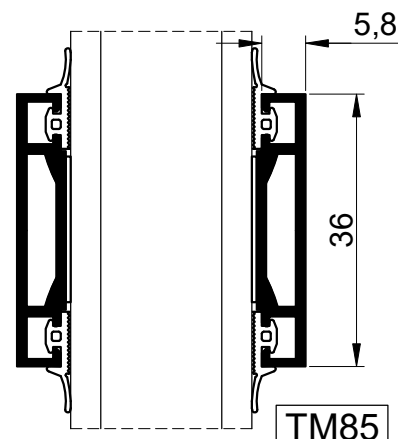
Ukрасna lajsna na staklu Decorative bar on the glass Декоративный переплет на стекле
