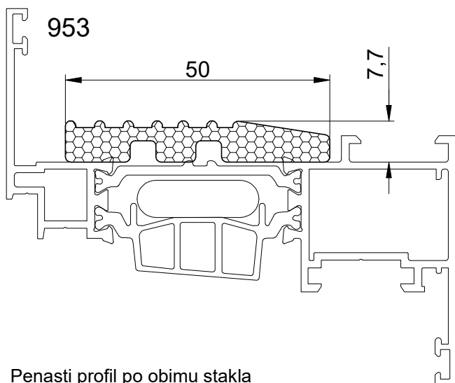
Penasti profil po obimu stakla Foam profile by glass girth Профиль пены по объему стекла
