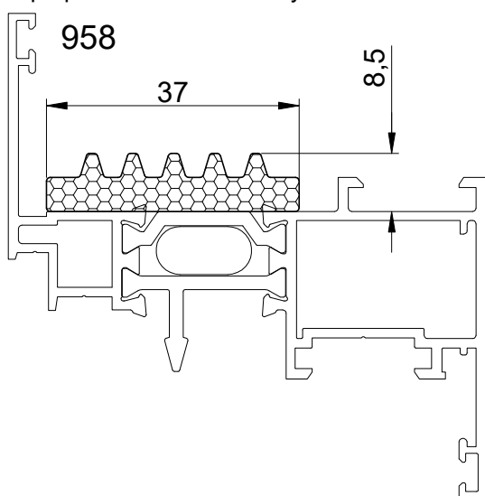
Penasti profil po obimu stakla Foam profile by glass girth Профиль пены по объему стекла
