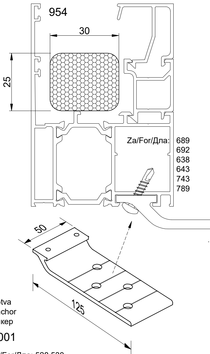
Penasti profil po obimu stakla Foam profile by glass girth Профиль пены по объему стекла
